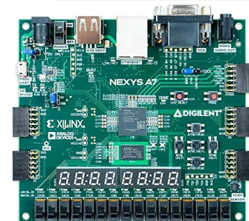
Nexys A7
